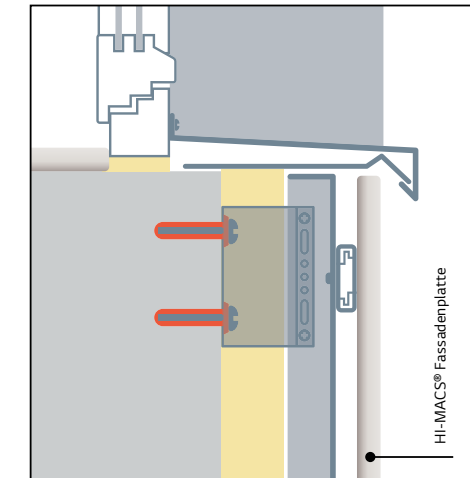
Fensterbrüstung
