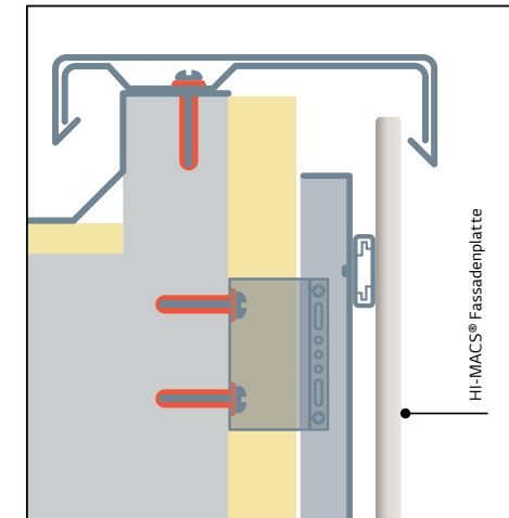
Attika-Abschluss (oberer Abschluss)
