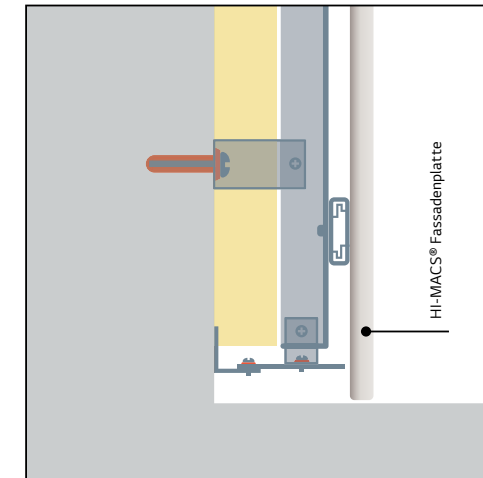
Sockel-Abschluss (unterer Abschluss)
